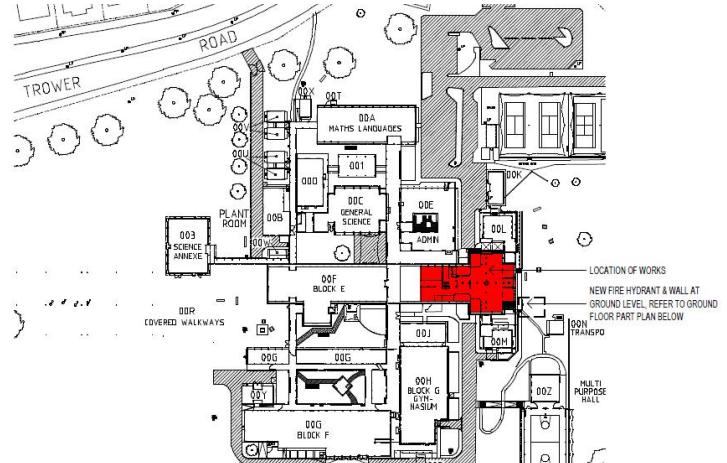
SITE PLAN 1:2000
